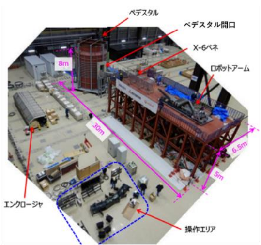
写真：櫛葉遠隔技術開発センター（JAEA）試験設備
