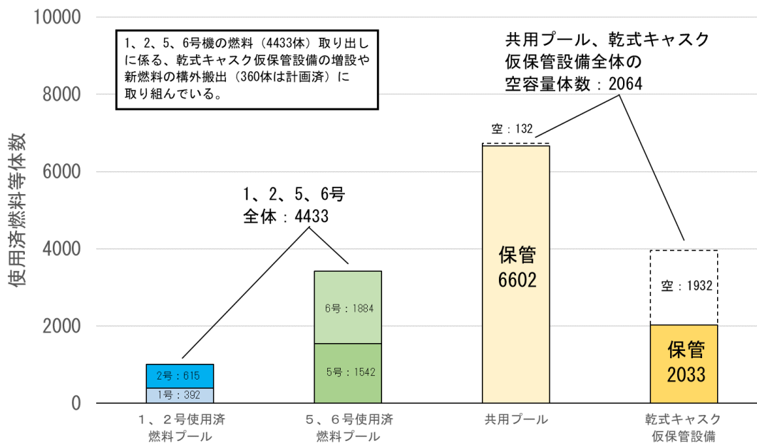
図 使用済燃料の保管状況（2022年5月時点）
