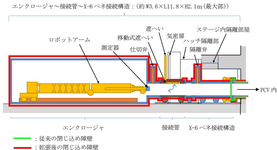
図 X-6 ペネ エンクロージャ等 構造概略図
