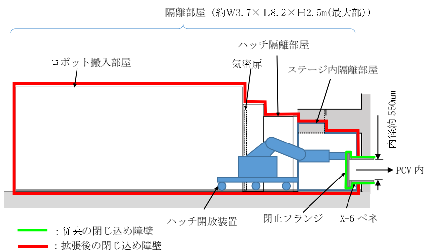
図 X-6 ペネ 隔離部屋 構造概略図
